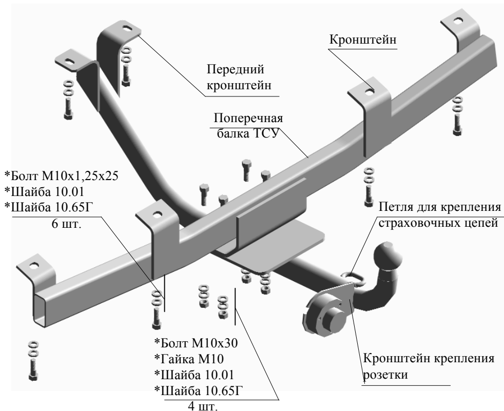
Рис.1 Тягово-сцепное устройство ТСУ 2123.Р (2123.02.Р)
