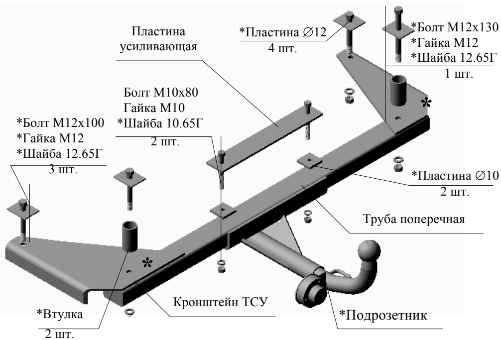
Рис.1 Тягово-сцепное устройство ТСУ 7410 ДЭУ.
