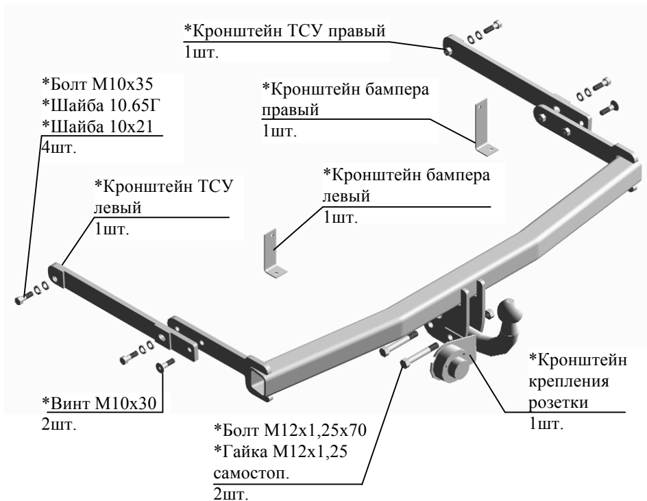
Рис.1 Тягово-сцепное устройство 6030
