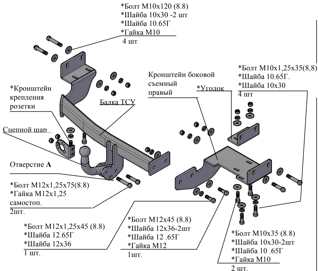
Рис.1 Тягово-сцепное устройство 7360
