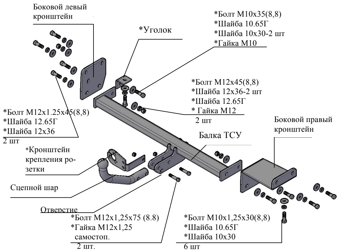
Рис.1 Тягово-сцепное устройство 7370.
