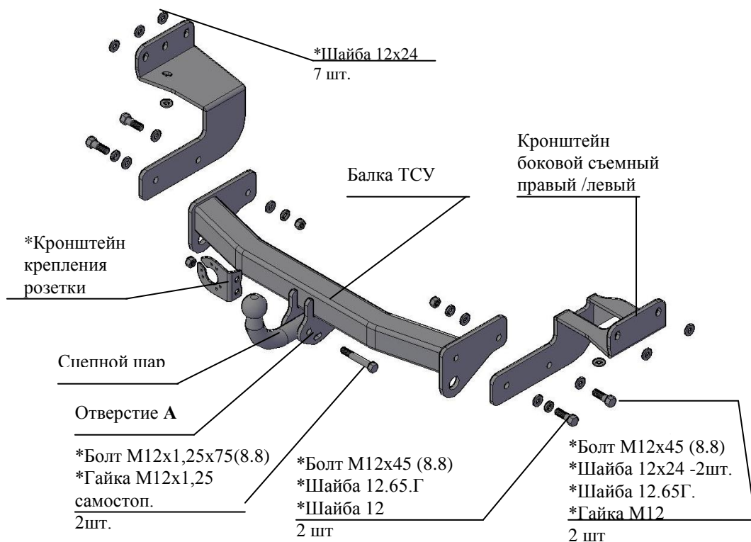
Рис.1 Тягово-сцепное устройство 7150
