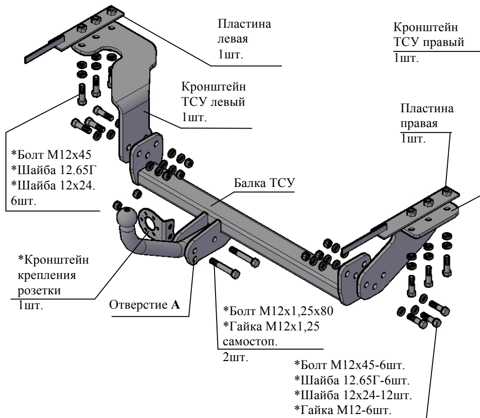
Рис.1 Тягово-сцепное устройство 7710
