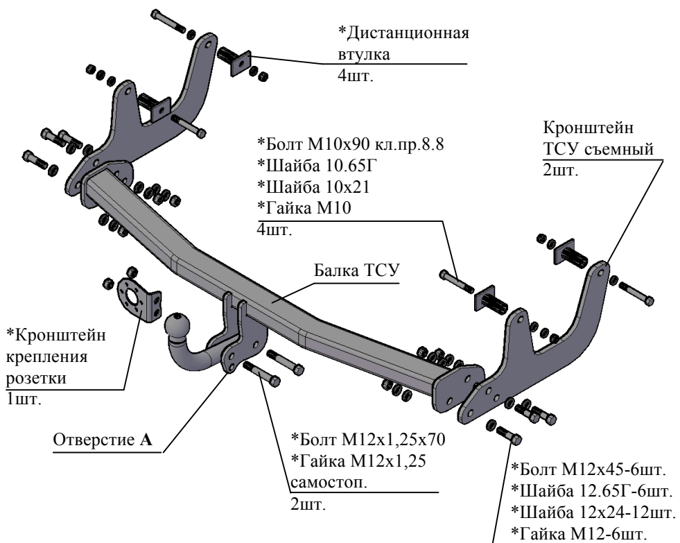
Рис.1 Тягово-сцепное устройство 9030
