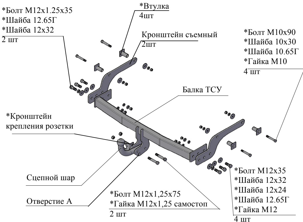
Рис.1 Тягово-сцепное устройство ТСУ 9031
