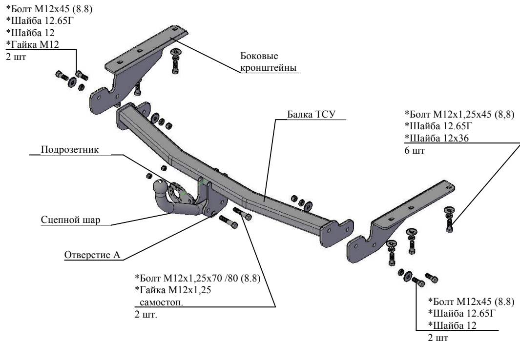
Рис.1 Тягово-сцепное устройство 7830.
