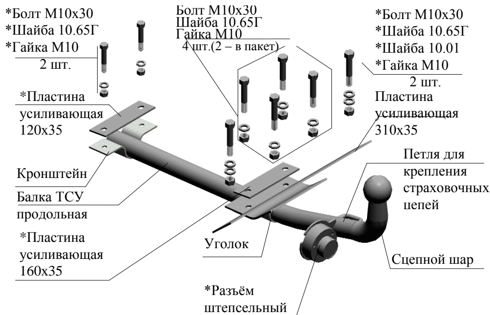
Рис.1 Тягово-цепное устройство ТСУ 1111
